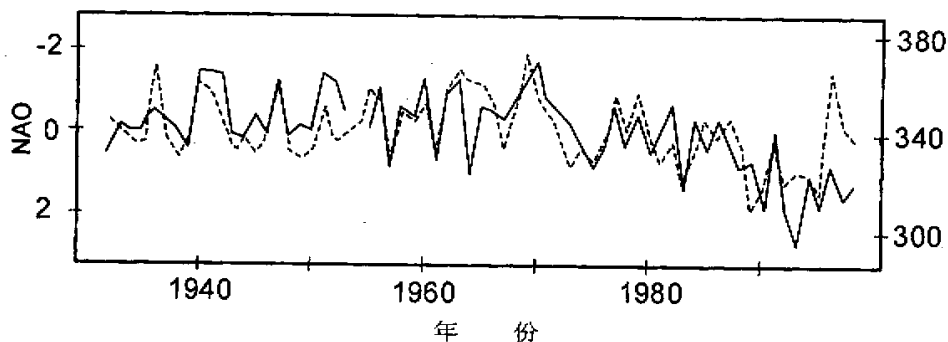
图 2 12~3 月瑞士阿罗萨站臭氧总量(实线)与 NAO 指数(虚线) [35]
