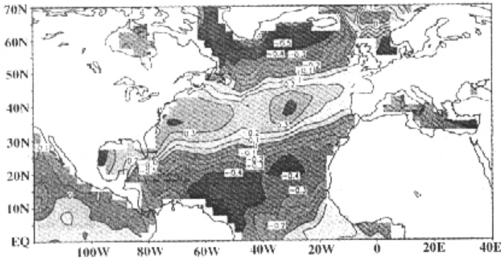
图3 实际观测资料中NAO与SST距平的相关系数分布 [53]
