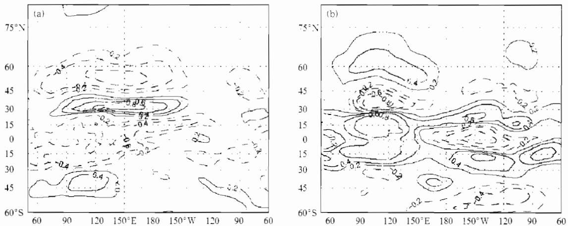
图 3 强度指数(a)和切变指数(b)与冬季 u_{200} 相关分布(图中阴影部分表示通过 95% 信度检验)
